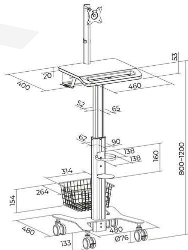
Soporte para escáner
