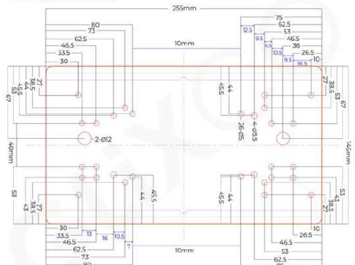
Plano de agujeros del plato (mm)
