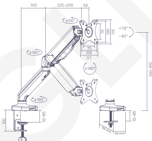
Sistema Gas Spring - Hidráulico
