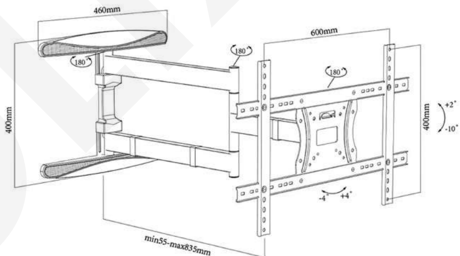
Brazo retraible
